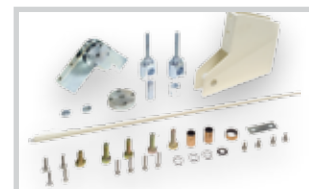
Kloubový kit pro zlomovací ráhna - max. výška stropu 3 m (pouze pro standardní obdel. ráhno)
