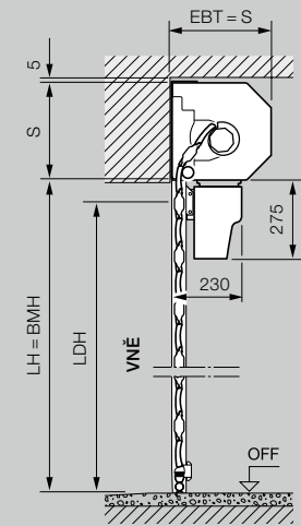
Rozsah velikostí vnitřních a venkovních rolovacích vrat
