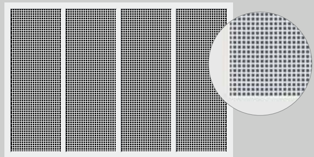
Motiv 413 a 433 Vnitřní výplň z perforovaného plechu s čtvercovými otvory, ventilační průřez 44,4 %
