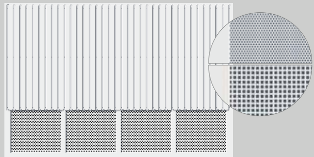
Motiv 414 Celoplošný ocelový vroubkovaný plech s výplň z perforovaného plechu s kruhovými nebo čtvercovými otvory, ventilační průřez 46,1 % (kruhové) resp. 44,4 % (čtvercové)
