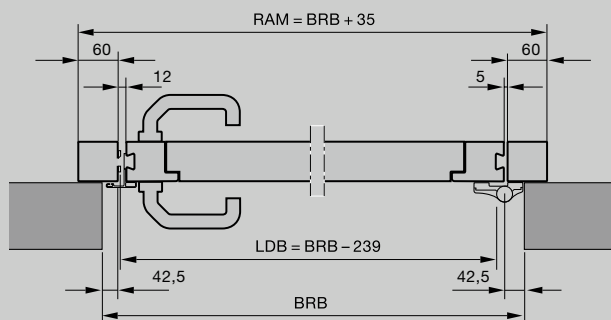
Montáž za otvorem
